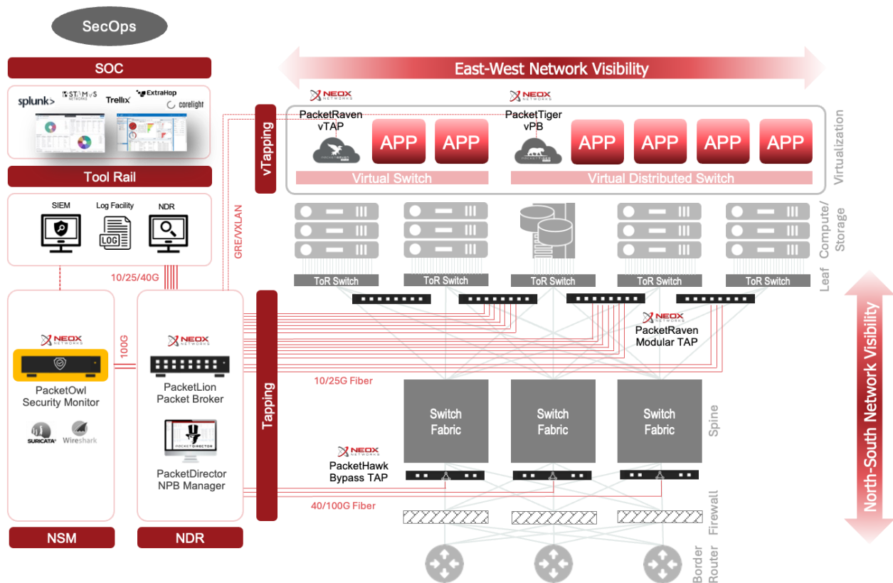
Diagramm-3: NEOX PacketOwl NSM Deployment im Rechenzentrum
